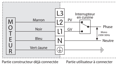
Schéma de câblage avec interrupteur va et vient
