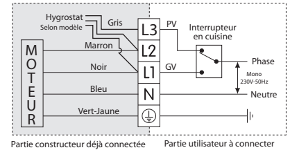
Schéma de câblage avec interrupteur va et vient
