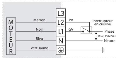
Schéma de câblage avec interrupteur
