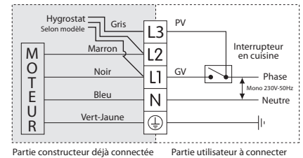
Schéma de câblage avec interrupteur
